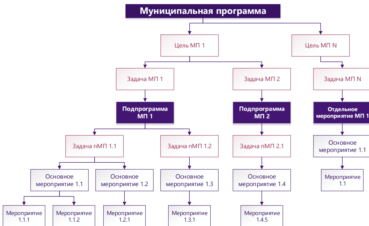
Рисунок 1 - Структура программы
